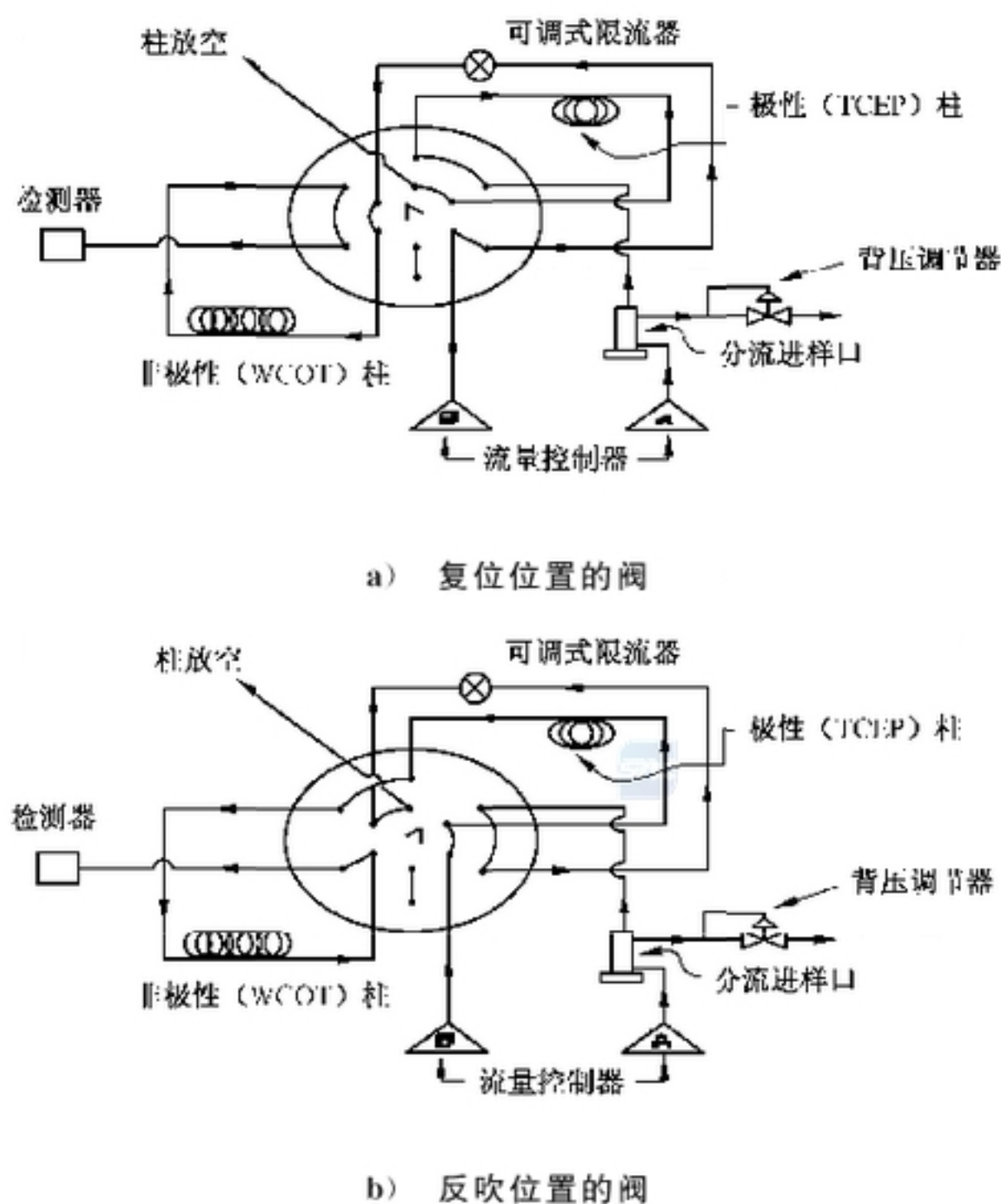
图 A.1 色谱系统示意图
