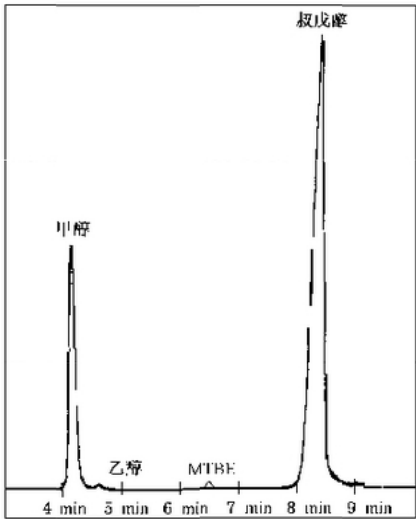
图 A.2 色谱结果示例
